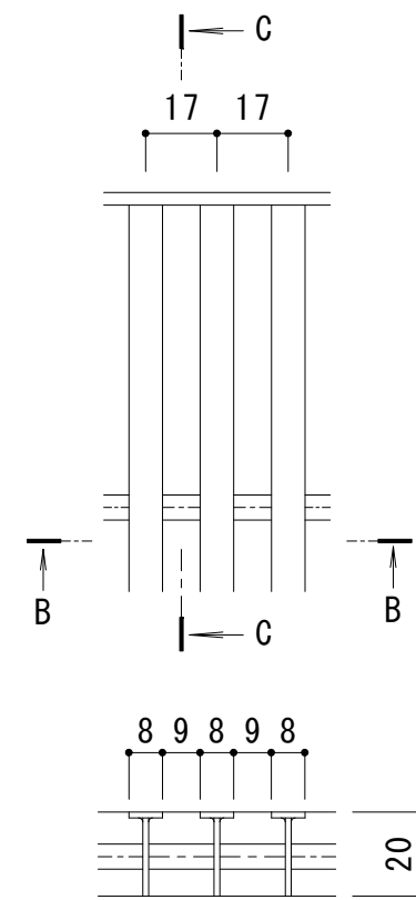
B-B断面図
