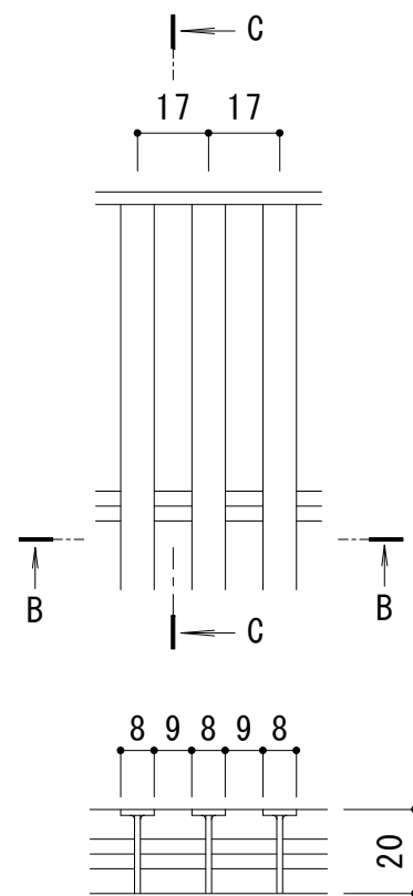
B-B断面図
