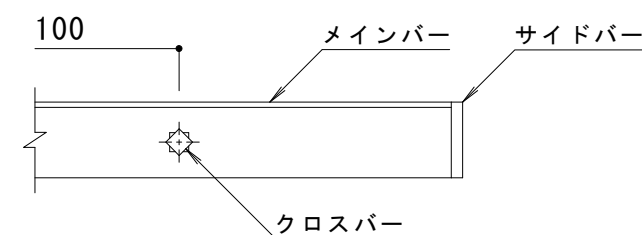
C-C断面図
