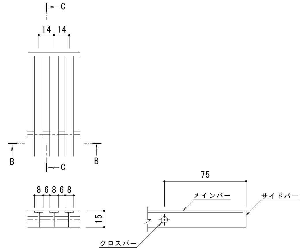
B-B断面図
