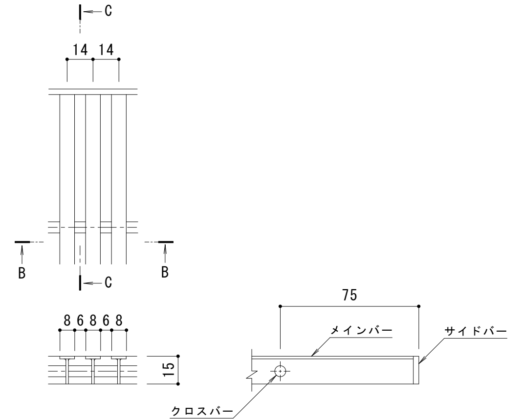
B-B断面図
