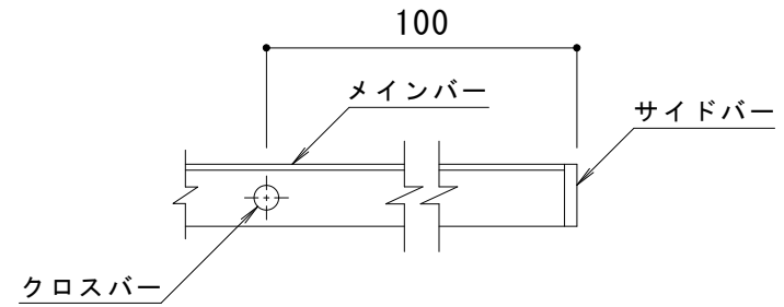
C-C断面図
