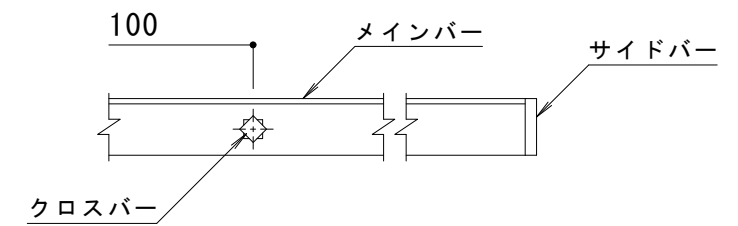
C-C断面図
