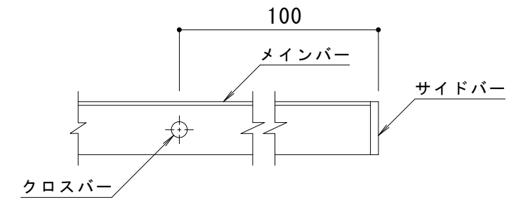
C-C断面図
