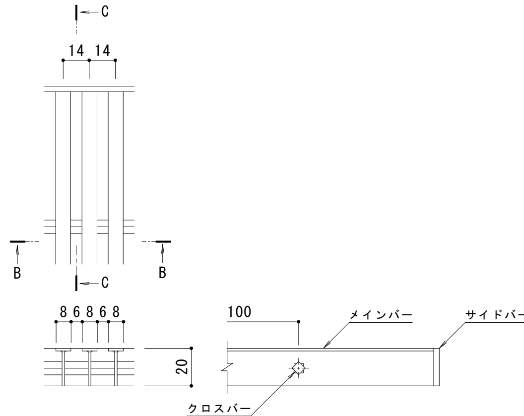
B-B断面図
