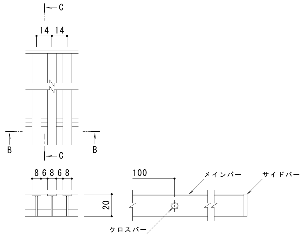
B-B断面図
