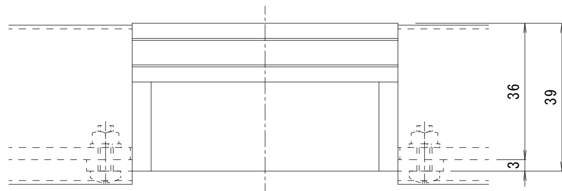
ラインプロテクターA 詳細図 S = 1 : 1
