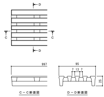
スリット蓋 詳細図 S=1:2
