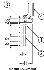
断面詳細図
