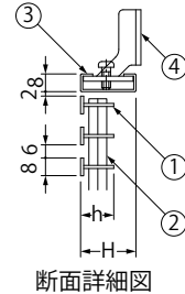
断面詳細図
