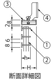
断面詳細図
