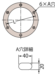
アンカーボルト取付寸法
