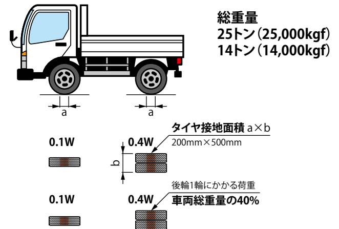
図1- T-25、T-14の荷重条件時の後輪1輪荷重と接地面積
