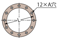
アンカーボルト取付寸法
