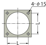
フックボルト取付寸法
