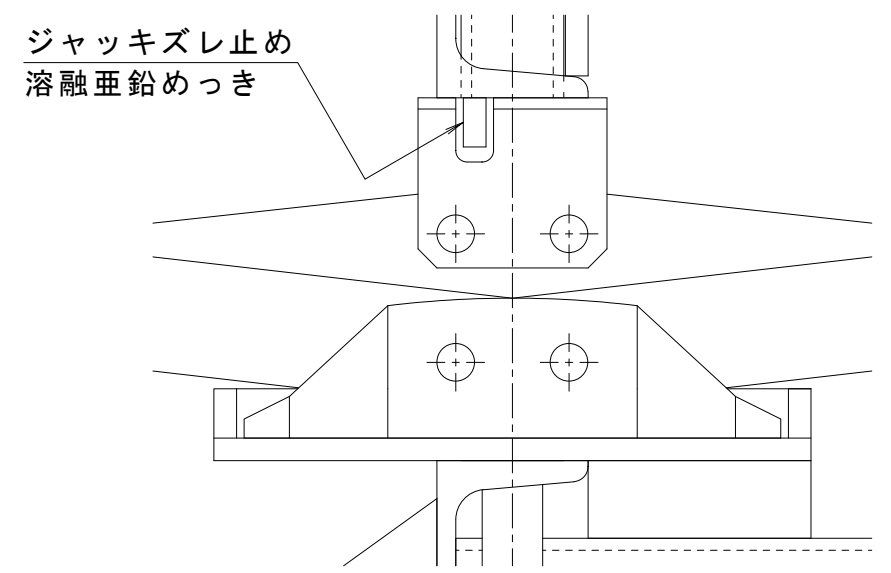
B-B 断面図 S = 1 : 2
