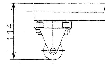
ハンドル部詳細 S=1:4
