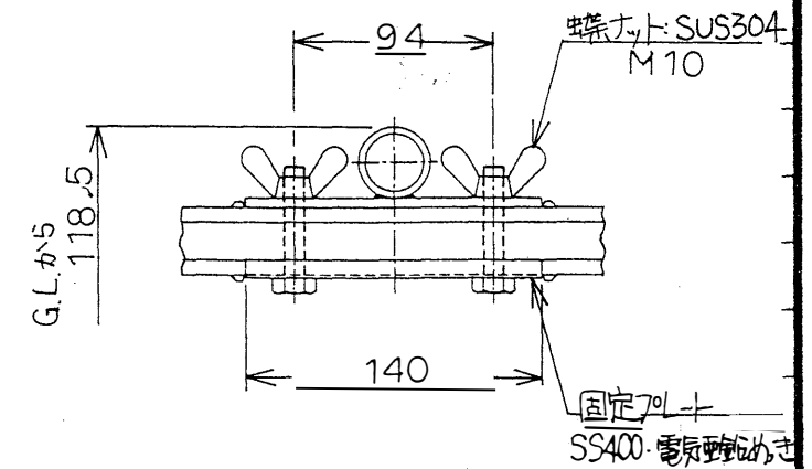
A-A断面詳細 S=1:4
