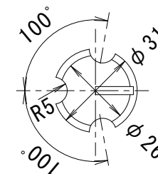
ロックボルト頭部詳細 S = 1 : 2
