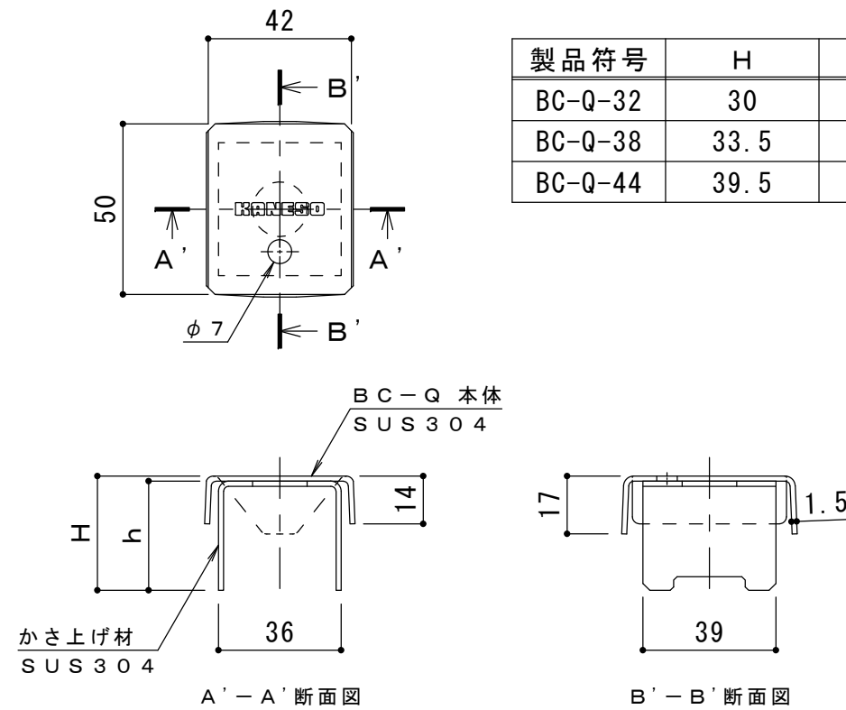
詳細図 S = 1 : 2
