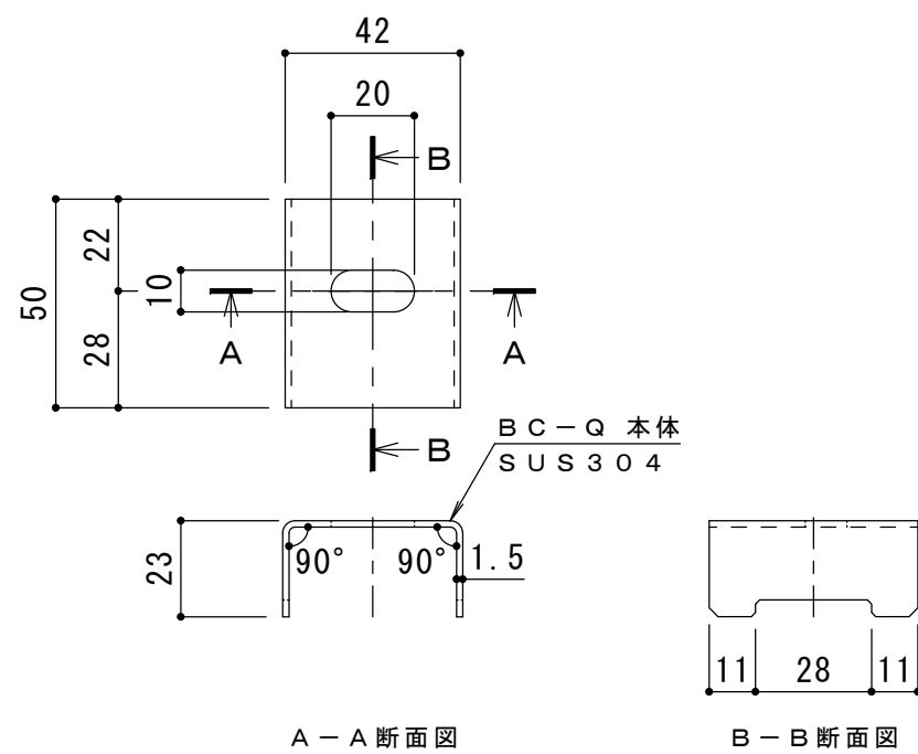
詳細図 S = 1 : 2
