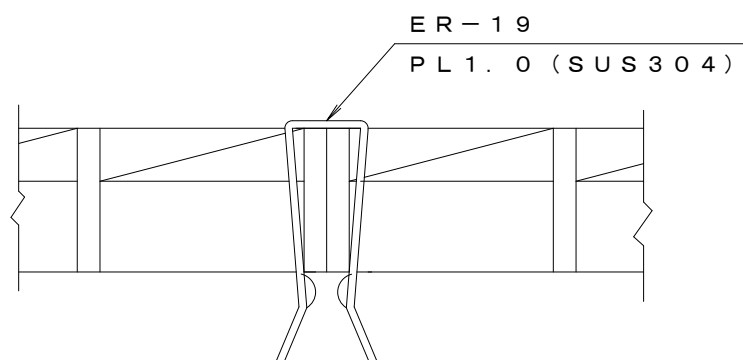
連結金具取付図
