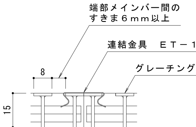
使用例 S = 1 : 1
