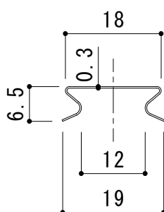
詳細図 S = 1 : 1
