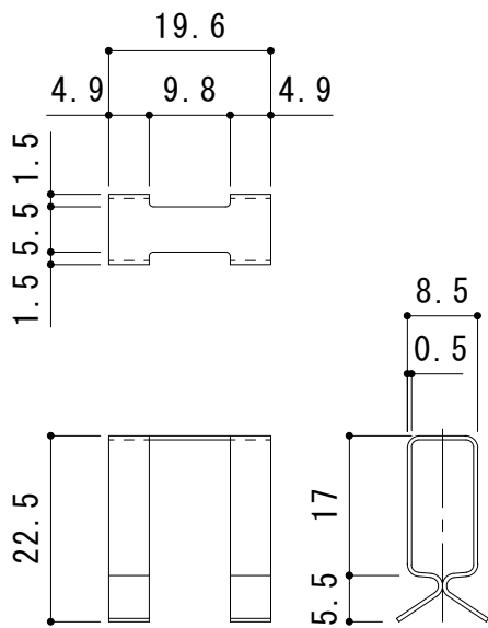
詳細図 S = 1 : 1
