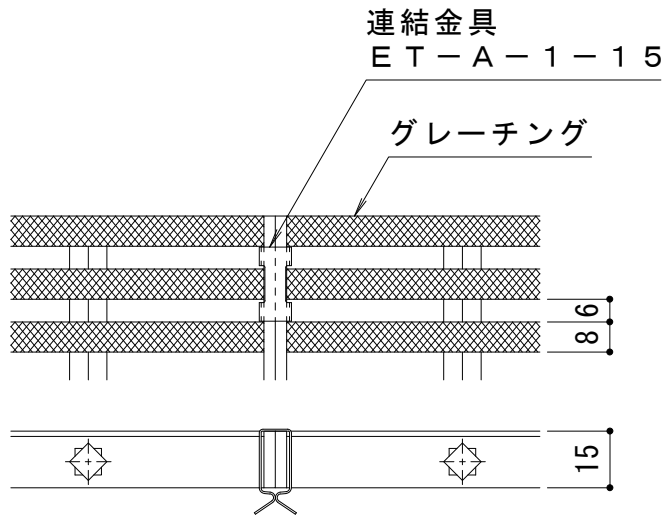
使用例 S = 1 : 2
