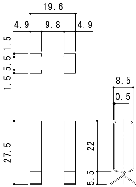
詳細図 S = 1 : 1
