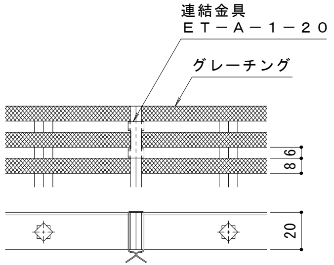
使用例 S = 1 : 2
