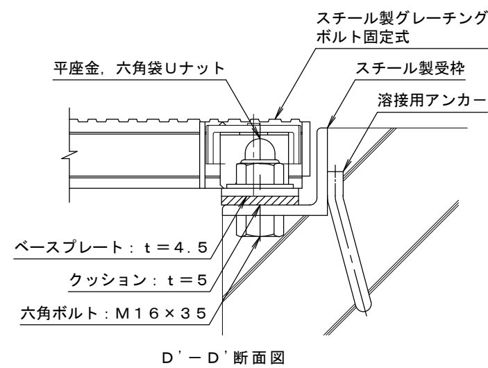
納まり参考図 S = 1 : 3
