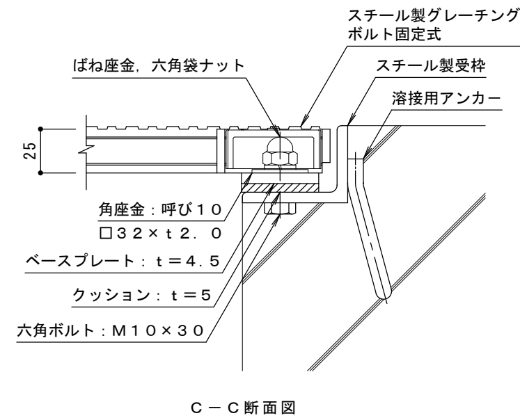
納まり参考図 S = 1 : 3
