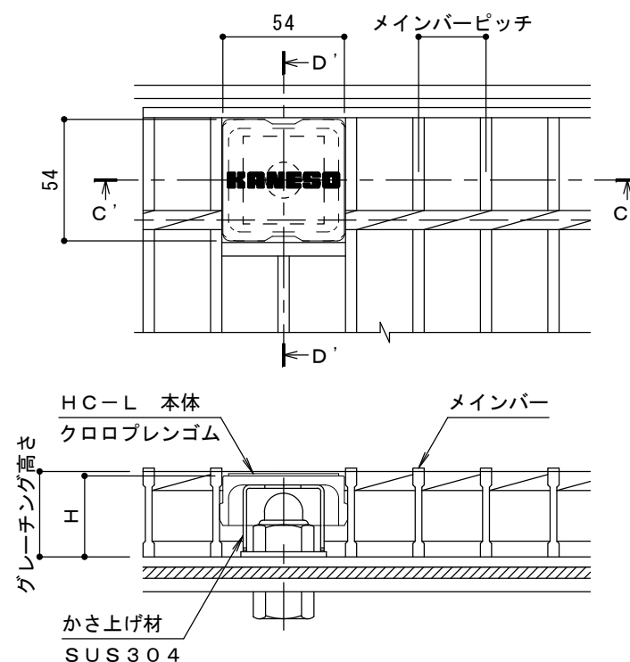
納まり参考図 S = 1 : 3
