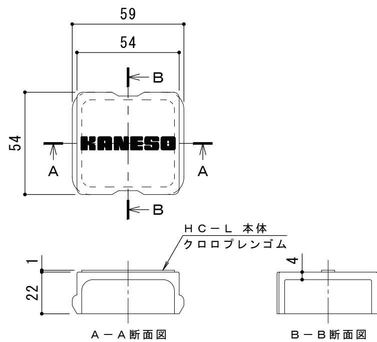
詳細図 S = 1 : 2
