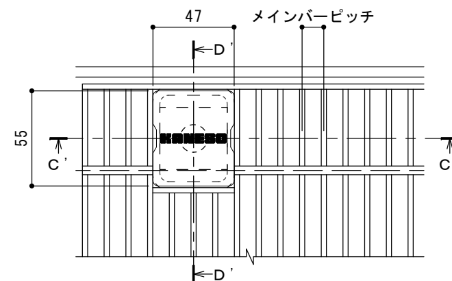
納まり参考図 S = 1 : 3
