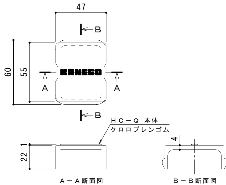
詳細図 S = 1 : 2
