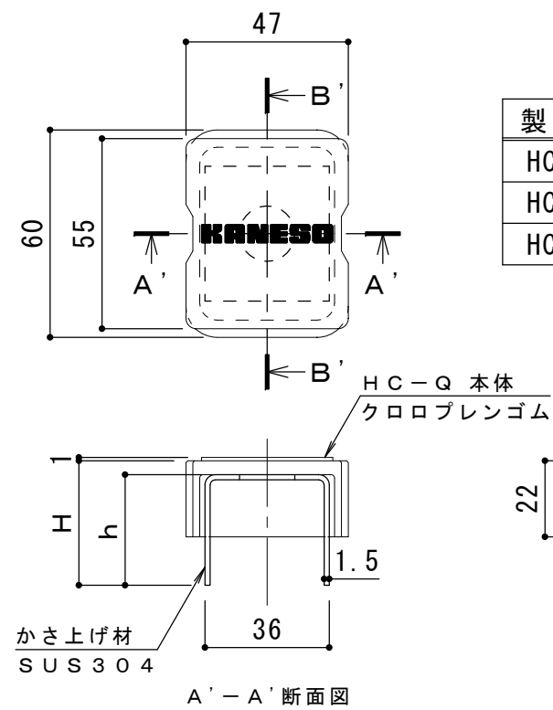
詳細図 S = 1 : 2
