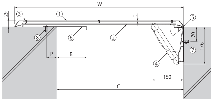
寸法・価格表 ステンレス製 Gタイプ:変位性能50%
