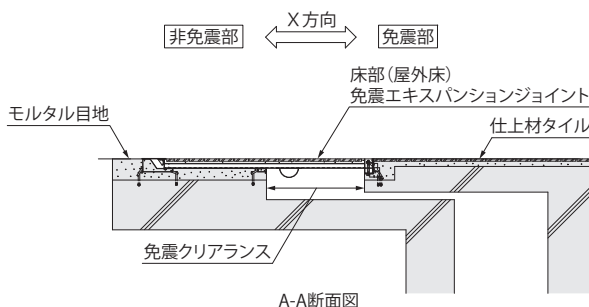
A-A断面図
