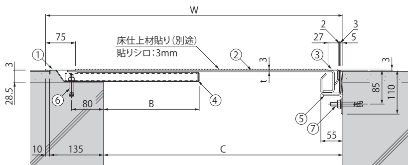
寸法・価格表 ステンレス製 Gタイプ:変位性能50%
