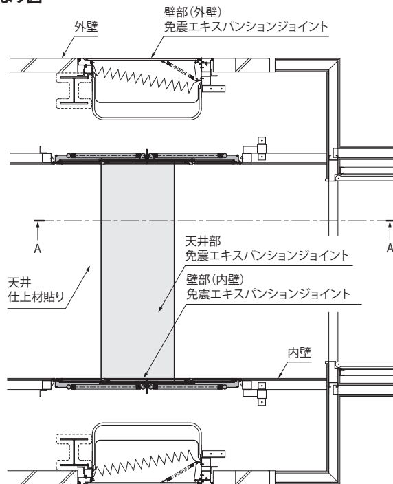
天井伏図
