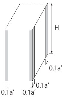
図3 壁部の部位
