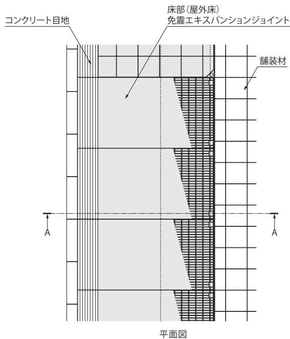
平面図
