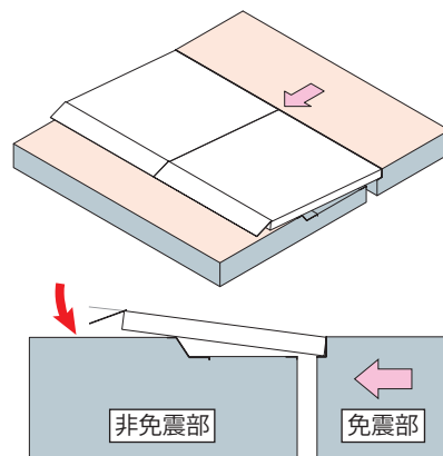
片側せり上がり式(床)・歩行者危害低減可動先端力バー
