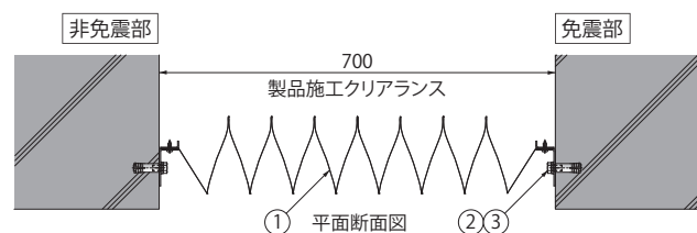
製品詳細図
