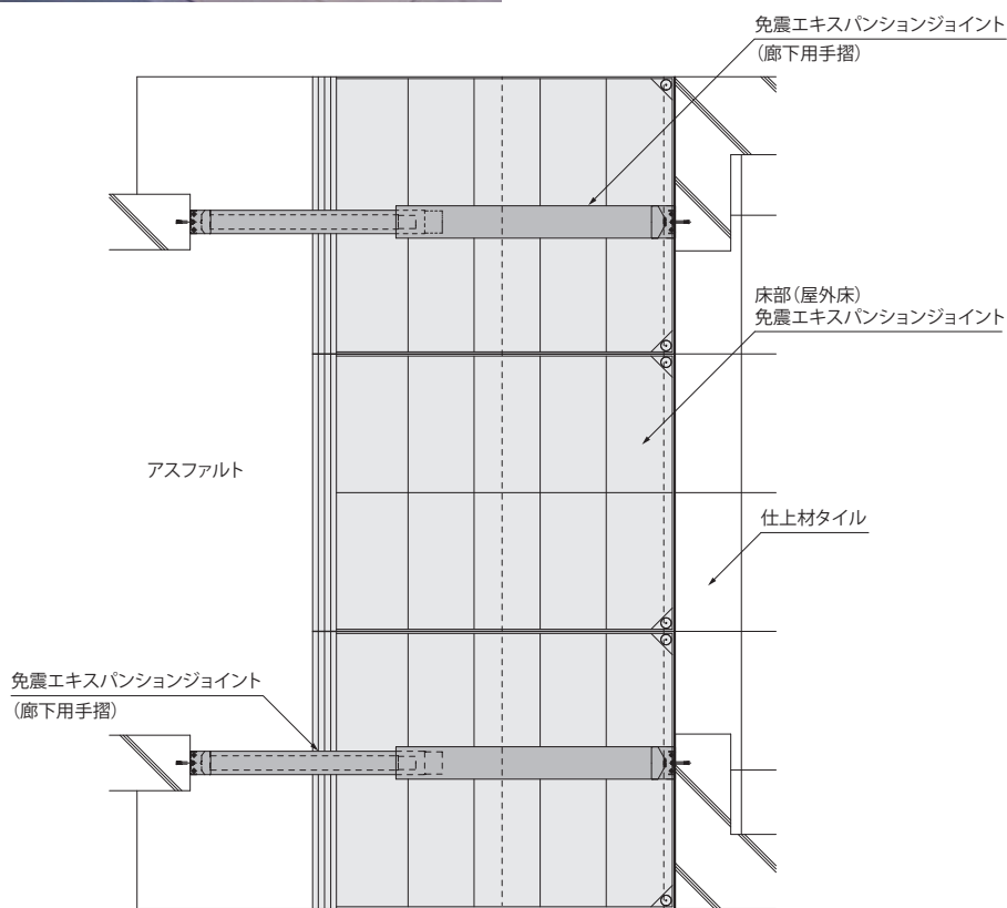
平面図
