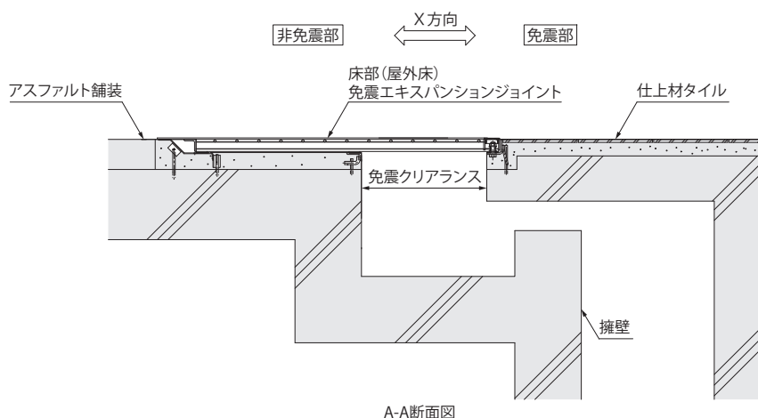
A-A断面図
