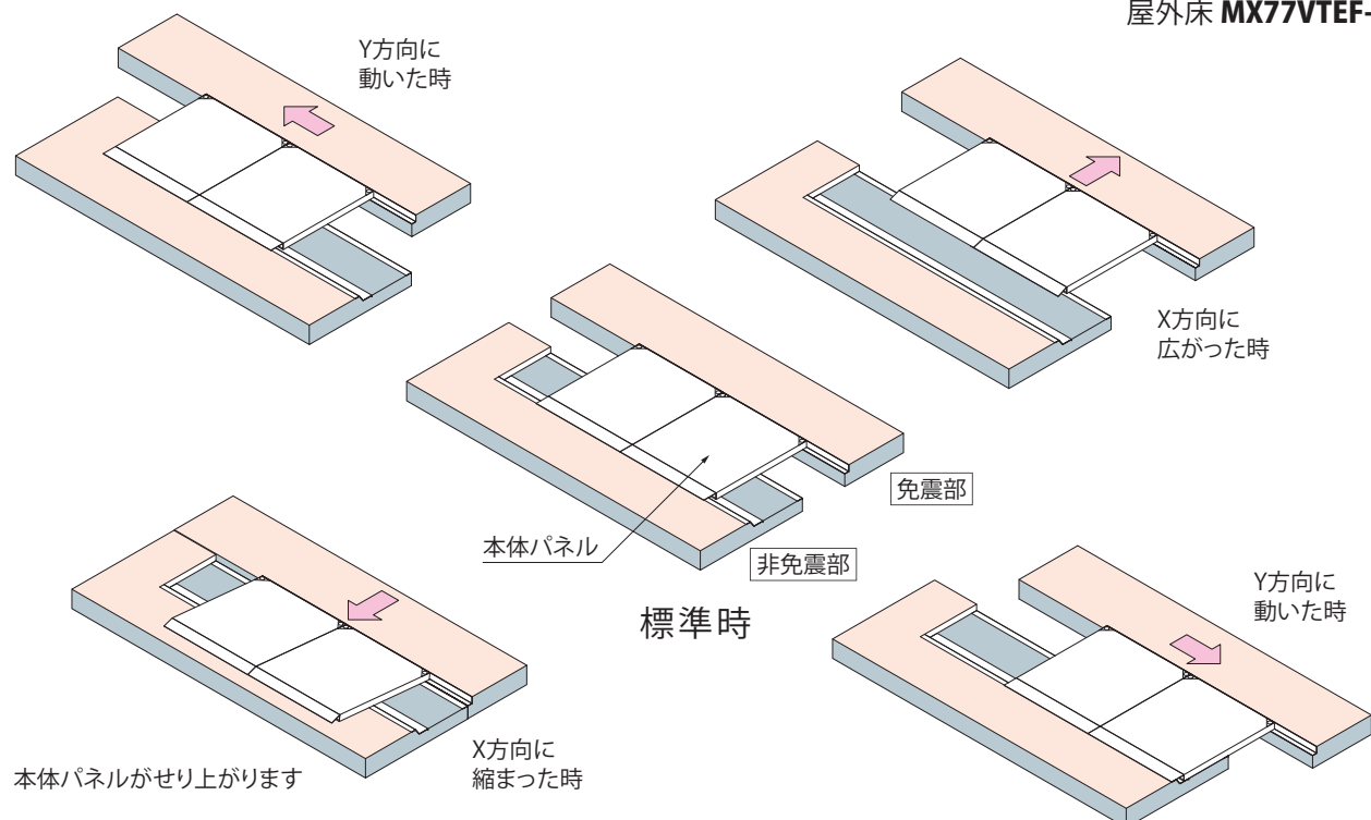
屋外床 MX77VTEF-U-M
