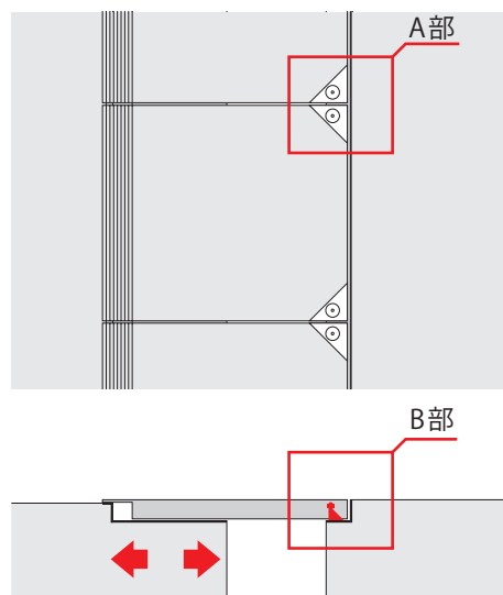
B部詳細図
