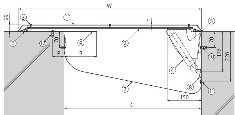
寸法・質量表 ステンレス製 Gタイプ:変位性能50%
