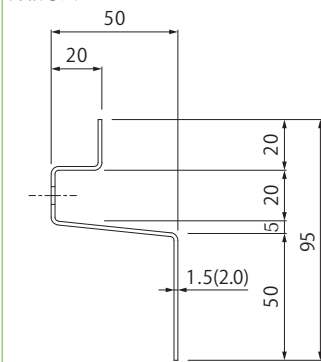
詳細寸法
