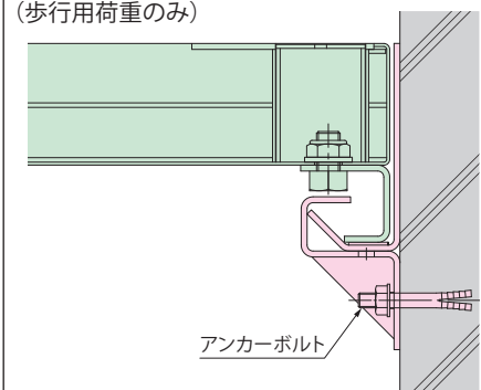
レールスライド受枠側面固定 (歩行用荷重のみ)
