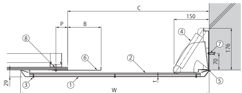
寸法・質量表 ステンレス製 Gタイプ:変位性能50%
