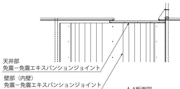
A-A断面図
