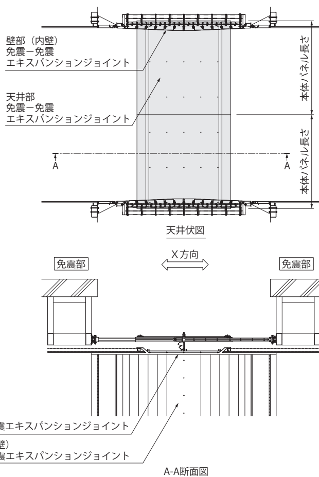
納まり図
