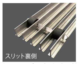
スリット裏側 クッションゴムが通行時の音鳴りを防止します。
