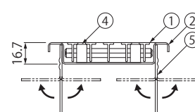
B-B断面図
