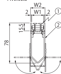
A-A断面図
