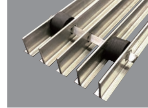
音鳴り防止 クッションゴム
