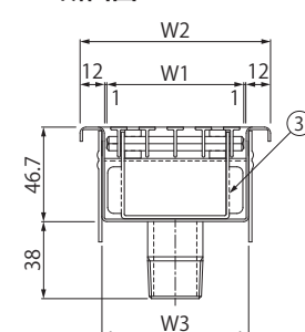
A-A断面図
