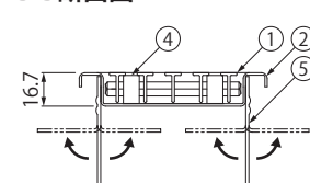
B-B断面図
