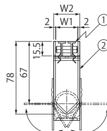
A-A断面図
