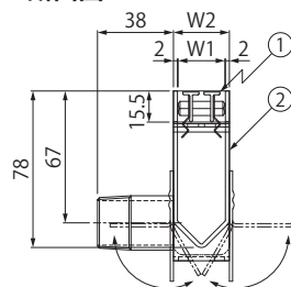
A-A断面図
