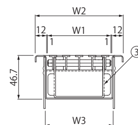
A-A断面図
