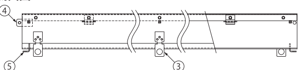
側面図
