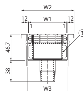
A-A断面図
