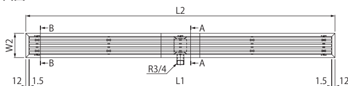
平面図
