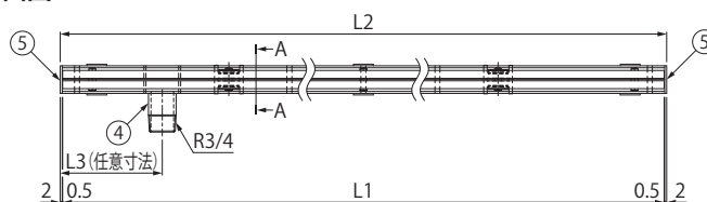
平面図
