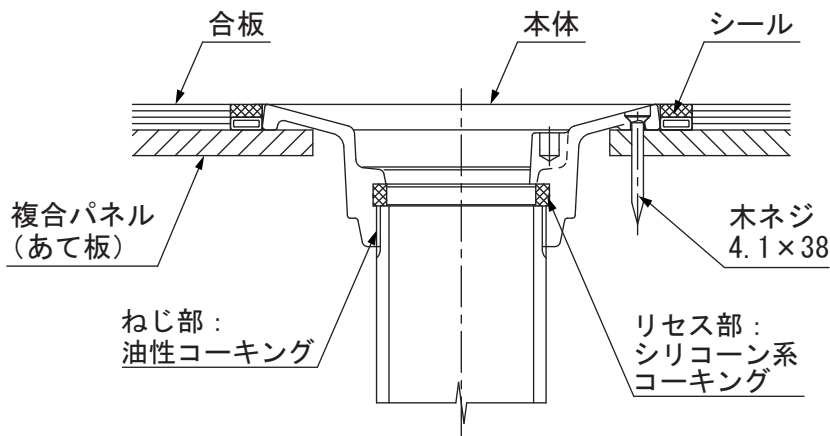
納まり図
