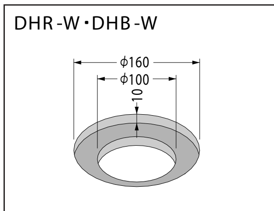
木下地加工寸法
