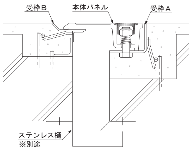
納まり図
