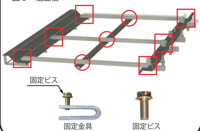
図c 組立後
