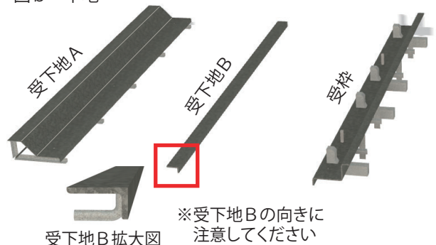
図b 下地
