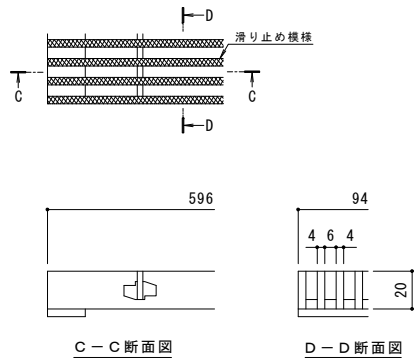
スリット蓋 詳細図 S = 1 : 2
