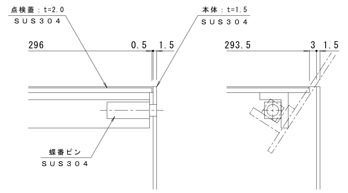
蝶番部 詳細 S = 1 : 1
