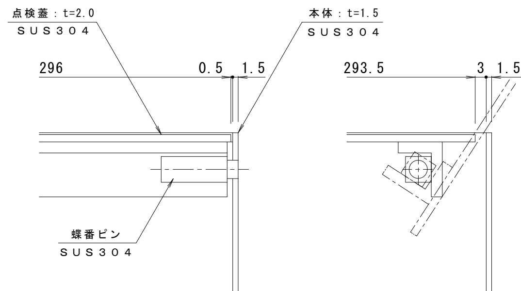
蝶番部 詳細 S = 1 : 1
