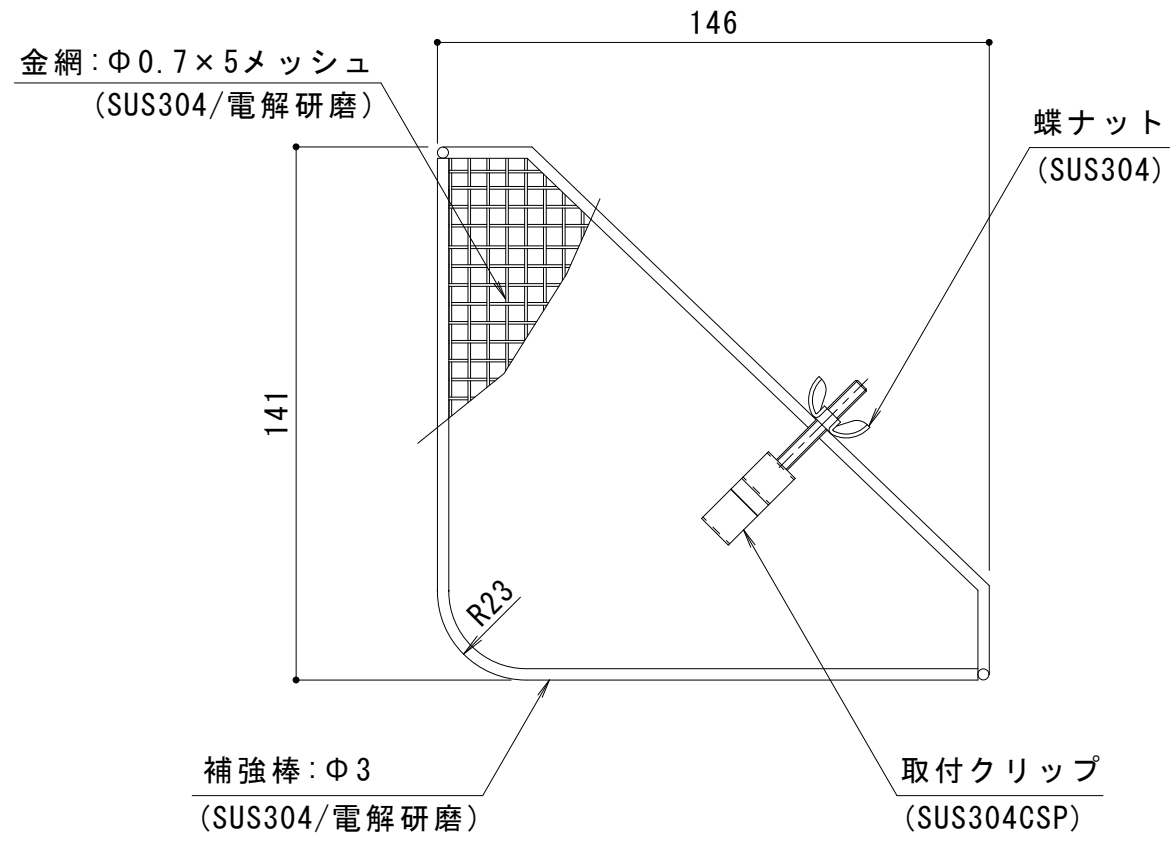
詳細図 S = 1 : 2
