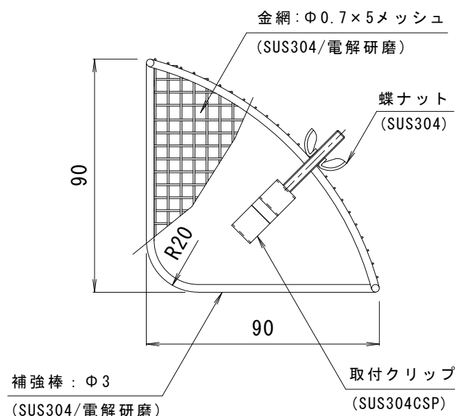
詳細図 S = 1 : 2
