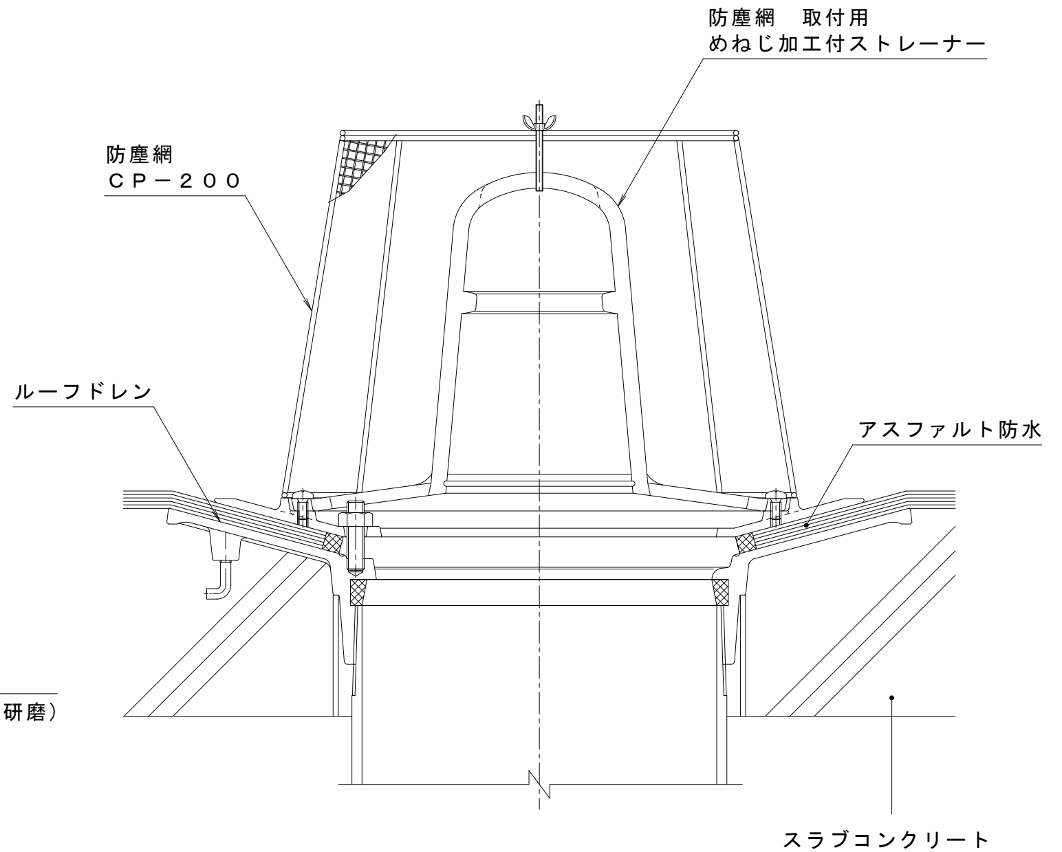
使用例 S = 1 : 3
