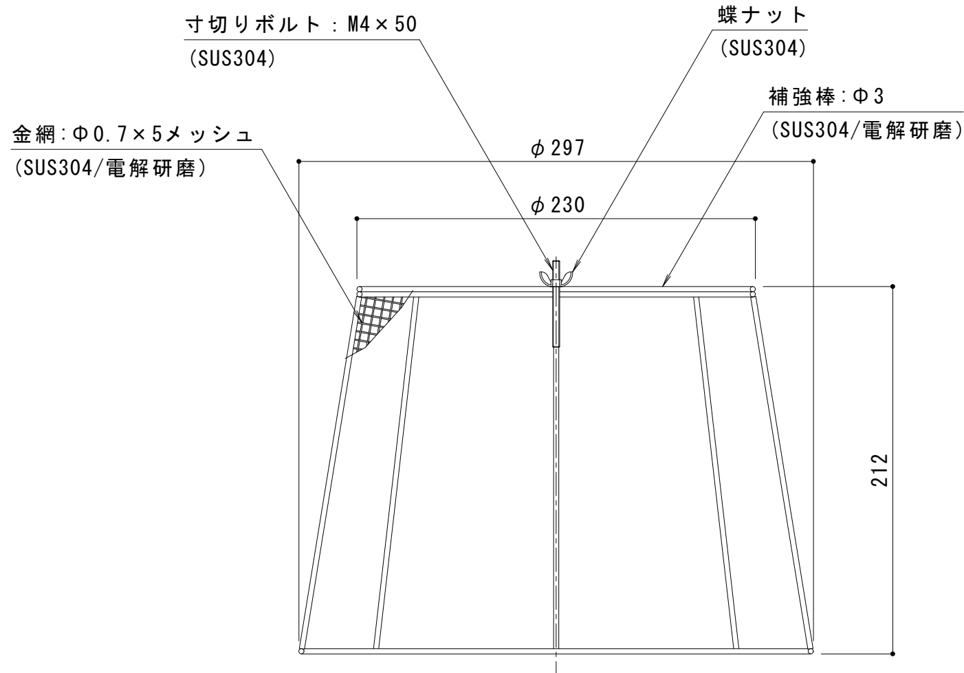
詳細図 S = 1 : 3
