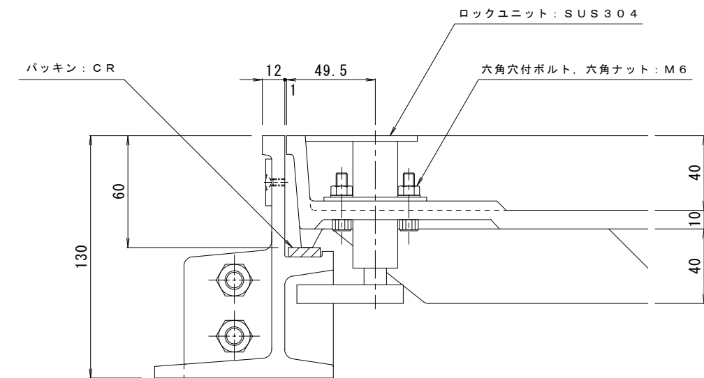
ロック部詳細図 S = 1 : 2
