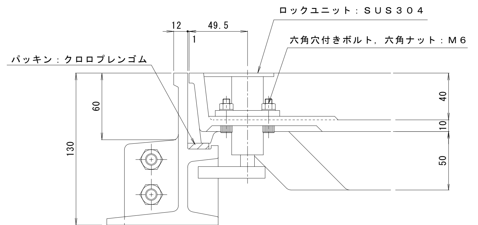
ロック部詳細図 S = 1 : 2
