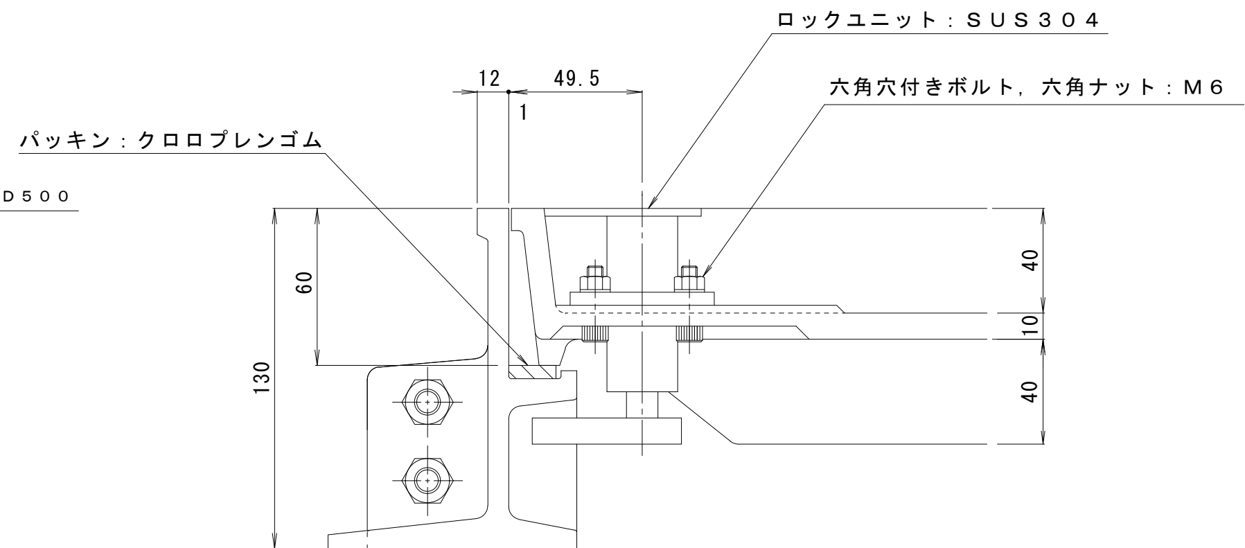
ロック部詳細図 S = 1 : 2
