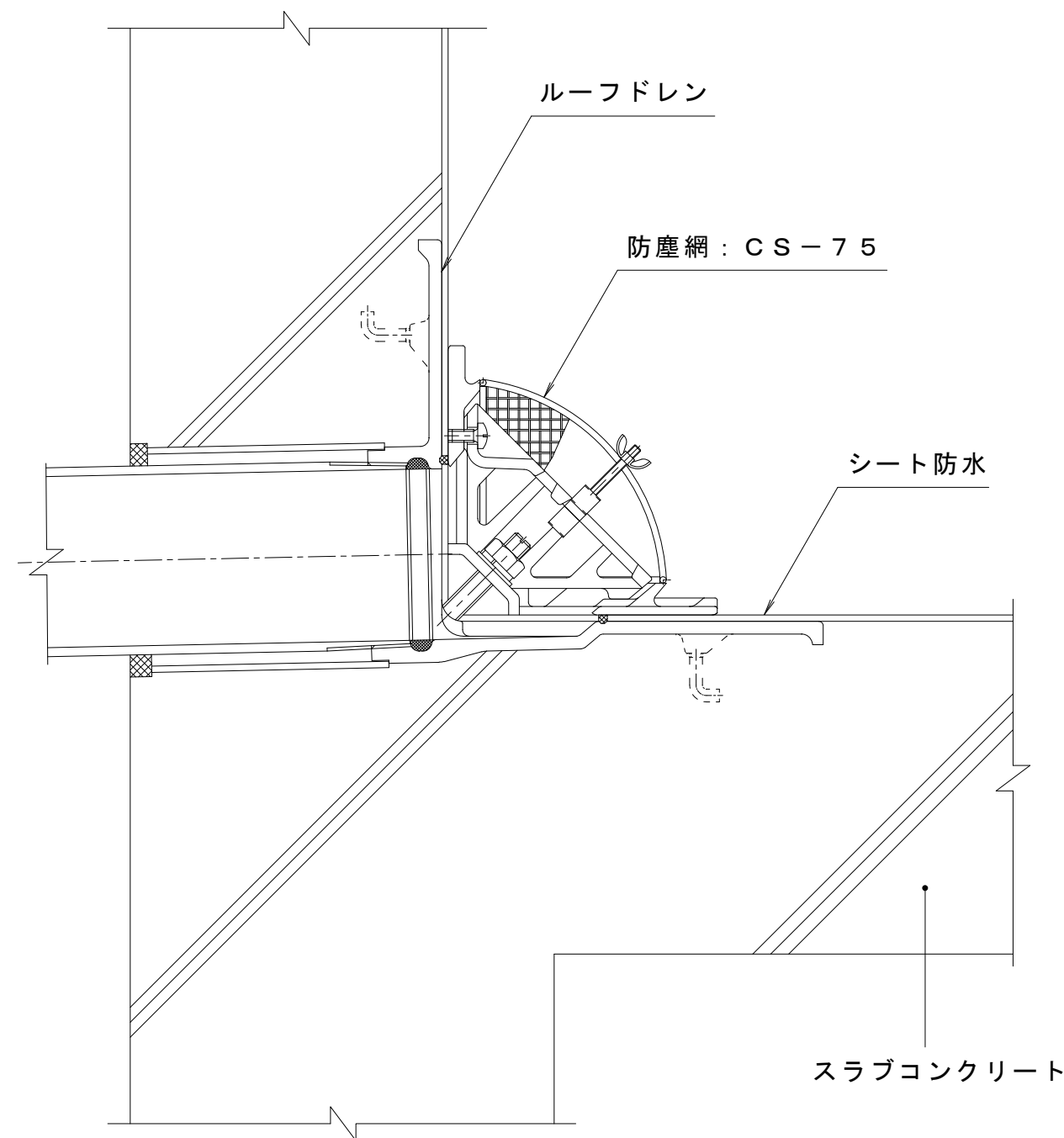
使用例 S = 1 : 3
