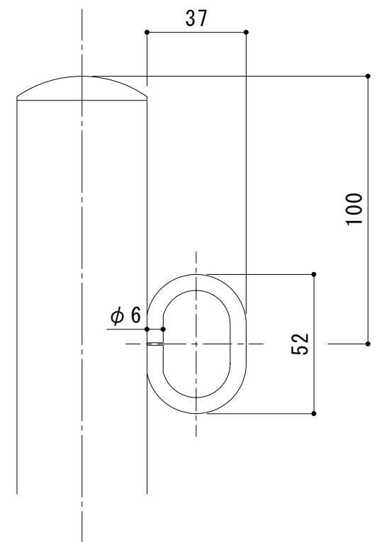
フック部詳細図 S = 1 : 2
