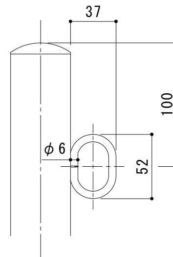
フック部詳細図 S = 1 : 3
