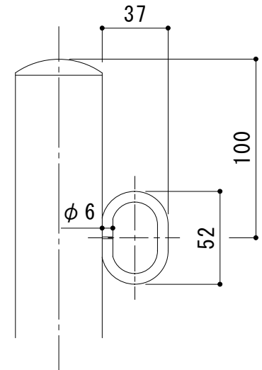
フック部詳細図 S = 1 : 3
