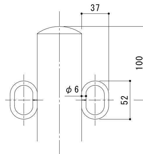
フック部詳細図 S = 1 : 3
