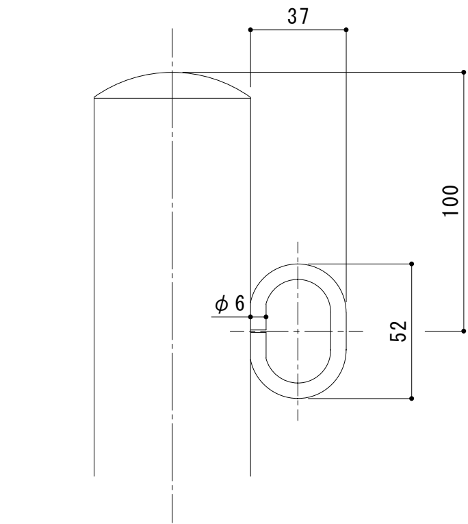
フック部詳細図 S = 1 : 2
