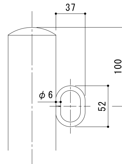
フック部詳細図 S = 1 : 3
