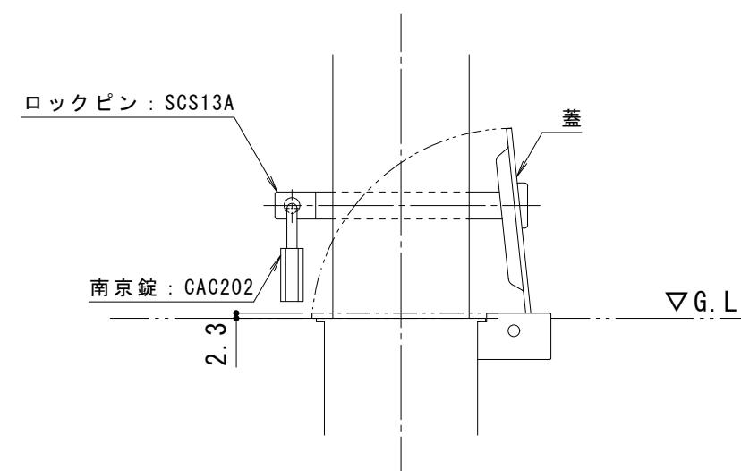
南京錠部詳細図 S = 1 : 3
