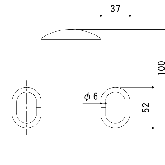
フック部詳細図 S = 1 : 3
