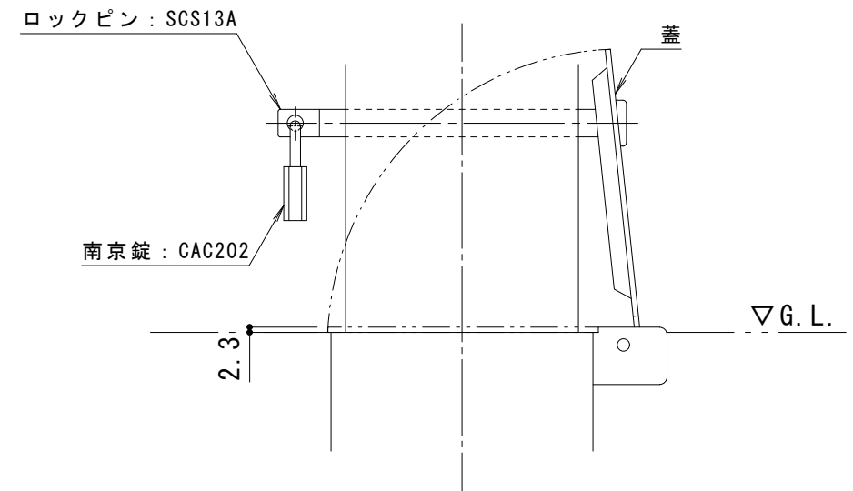
南京錠部詳細図 S = 1 : 3
