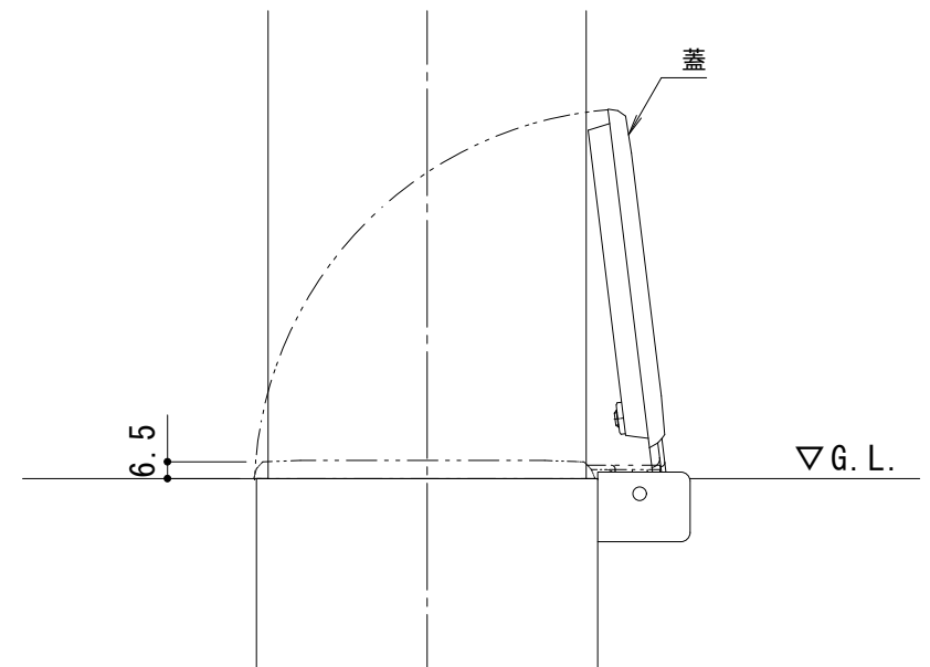
埋設管蓋部詳細図 S = 1 : 3
